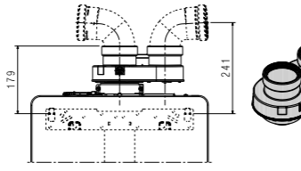
CONDOTTI SDOPPIATI Ø 80-80
