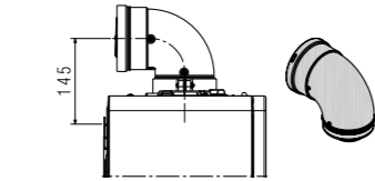
CONDOTTO COASSIALE Ø 60-100
