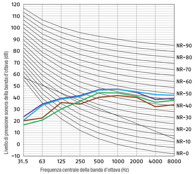
RAFFRESCAMENTO A35W7
