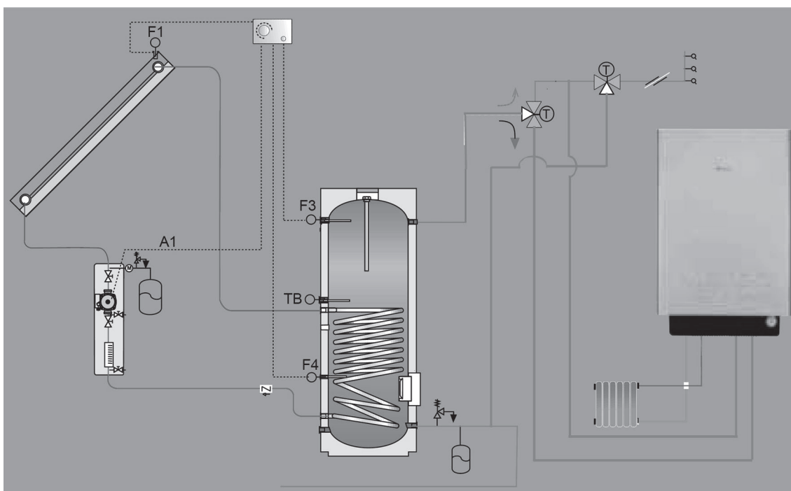
Schema di funzionamento: sistema solare a circolazione forzata, abbinato a caldaia murale combinata a condensazione.
