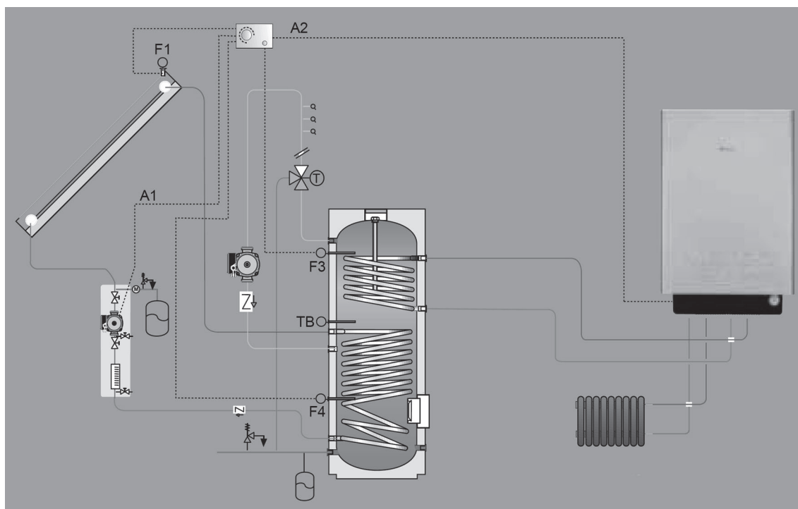
Schema di funzionamento: sistema solare a circolazione forzata, abbinato a caldaia murale solo riscaldamento a condensazione.
